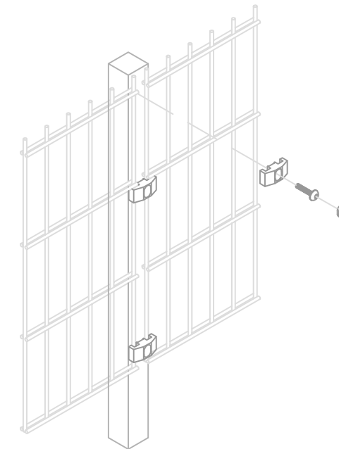
2 FINAL ASSEMBLY ISOMETRIC SK1 SCALE: N.T.S.
