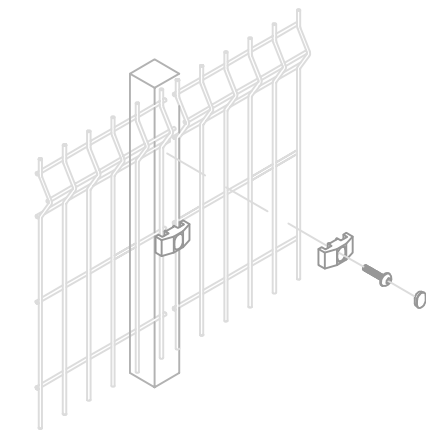
2 FINAL ASSEMBLY ISOMETRIC SK1 SCALE: N.T.S.
