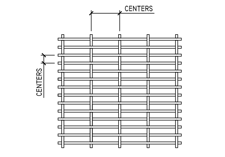
2 SELECT STYLE 1000 AI RETANGULAR WEAVE MESH SCALE: 3"=1'-0"
