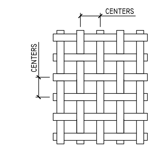
6 SELECT STYLE 3000 AI FLAT BASKET WEAVE MESH SCALE: 3"=1'-0"
