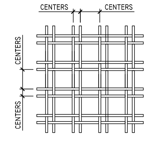
5 SELECT STYLE 2500 AI SQUARE DOUBLE WEAVE MESH SCALE: 3"=1'-0"
