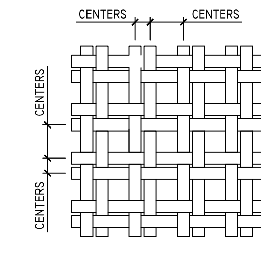
7 SELECT STYLE 3500 AI FLAT BASKET DOUBLE WEAVE MESH SCALE: 3"=1'-0"
