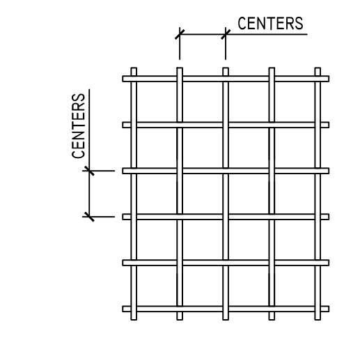
4 SELECT STYLE 2000 AI SQUARE WEAVE MESH SCALE: 3"=1'-0"
