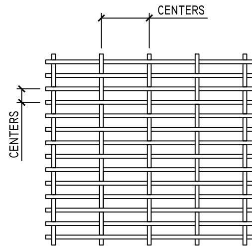
1 SELECT STYLE 1000 SK1 SCALE: 3"=1'-0"
