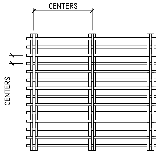
2 SELECT STYLE 1500 SK1 SCALE: 3"=1'-0"
