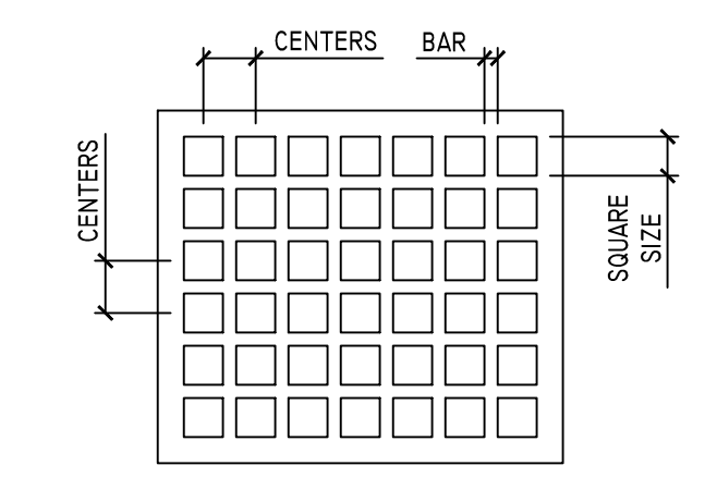
4 STANDARD SQUARE HOLES AI SCALE: 3"=1'-0"
