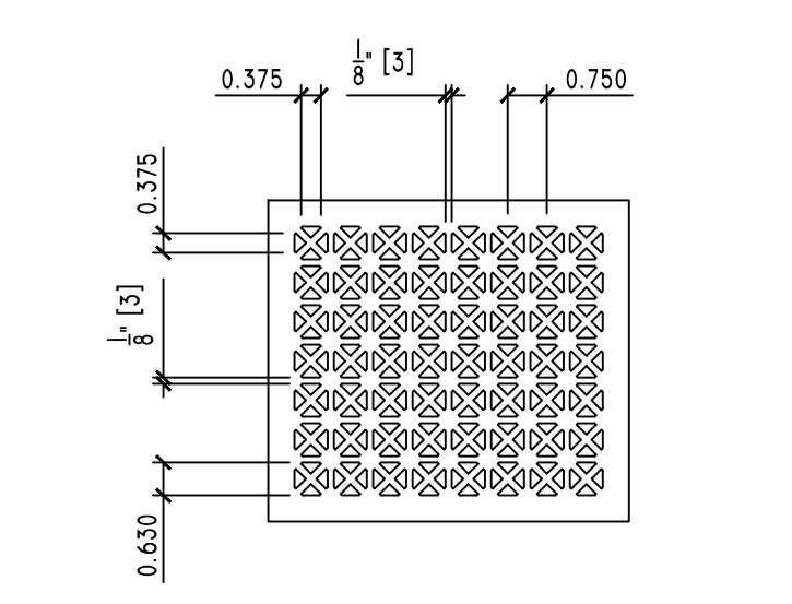
9 GRECIAN DECORATIVE AI SCALE: 3"=1'-0"
