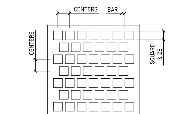
5 STAGGERED SQUARE HOLES AI SCALE: 3"=1'-0"
