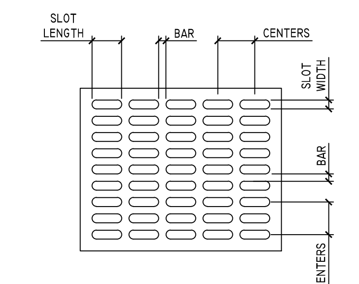
6 STANDARD SLOTTED HOLES AI SCALE: 3"=1'-0"
