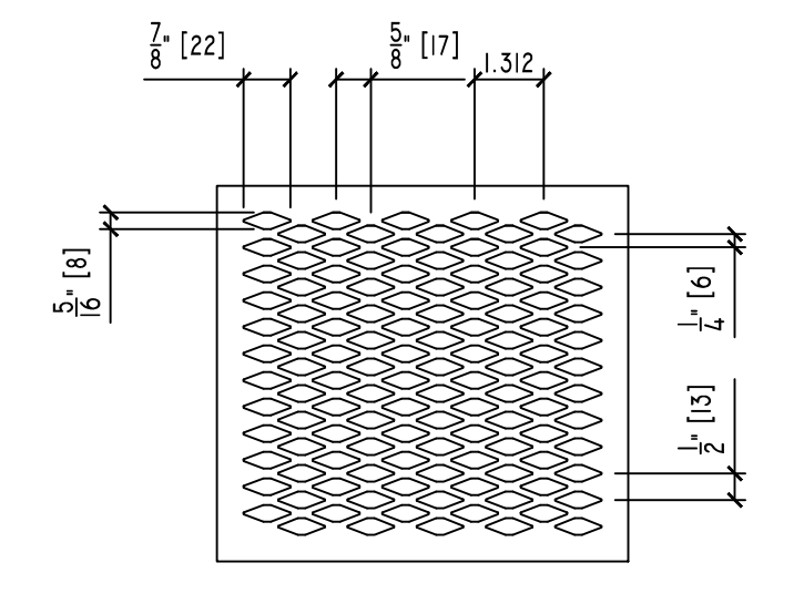
11 DIAMOND STAGGERED DECORATIVE AI SCALE: 3"=1'-0"
