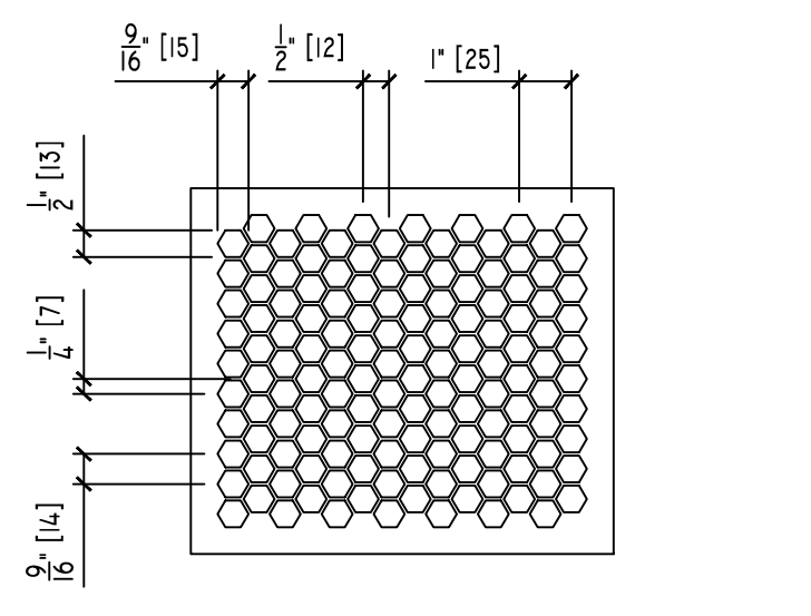
8 HEXAGONAL DECORATIVE AI SCALE: 3"=1'-0"
