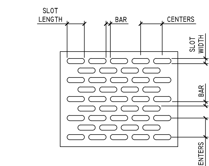
7 STAGGERED SLOTTED HOLES AI SCALE: 3"=1'-0"
